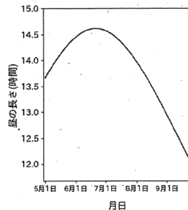
図2 つくば市における昼の長さ
